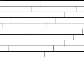
Pravilno polaganje pločica (smicanje na 1/5 dužine)
